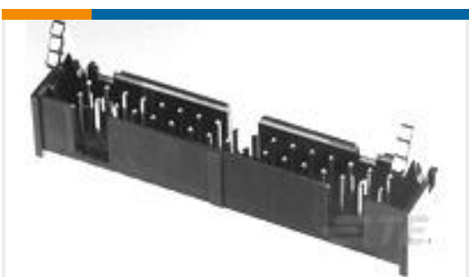
TE 产品编号1761606-8 IDC LOW PRO HDR 24P VERT LG LA
