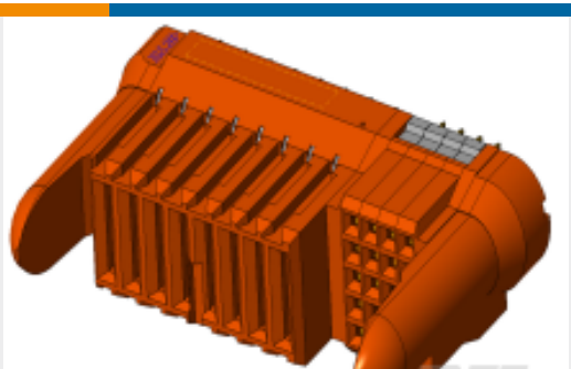
TE 产品编号1892787-9 Assy Vert MINIPAK HDL Rcpt 20s
