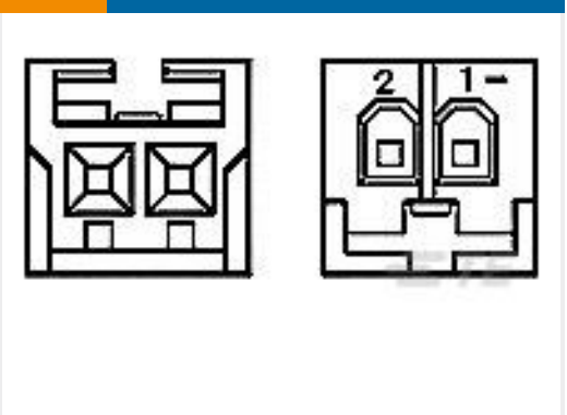
TE 产品编号172486-2 2P REC HSG CRIMP EI SER
