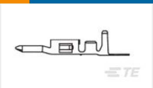
TE 产品编号794955-3 VAL-U-LOK PIN PHBZ SN 22-18AWG
