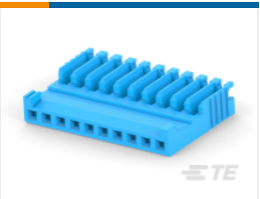
TE 产品编号1-281786-2 HE13/HE14 IDC 母端，SRST，AWG24-2
