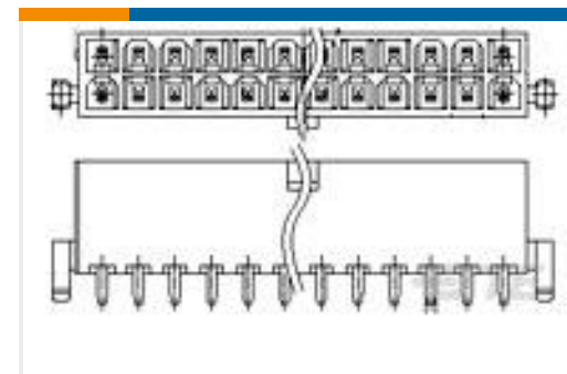
TE 产品编号2-1775099-1 ATX PWR CONN 2 BDLK 6 POS
