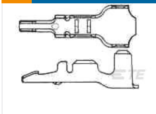
TE 产品编号170197-1 MINI AMP-IN 24-20 AWG
