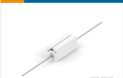
TE 产品编号1-1623742-0 线绕电阻器：轴向安装，17 瓦特
