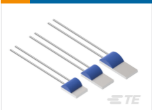
TE 产品编号NB-PTCO-032 RTD 铂金薄膜元件
