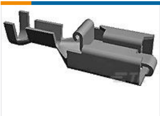
TE 产品编号160831-4 PL REC 1.0-2.5 MM2 .0160 X 2.060 TPPHBZ
