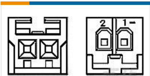
TE 产品编号172486-2 2P REC HSG CRIMP EI SER
