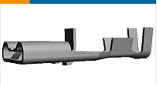
TE 产品编号170328-1 250 PL MKII REC. 18-14AWG PTBR
