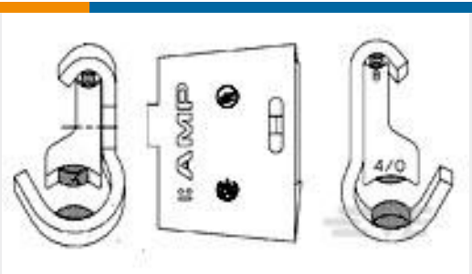
TE 产品编号83623-9 MINIWEDGE,LRG SL,4/0-#10,12,14
