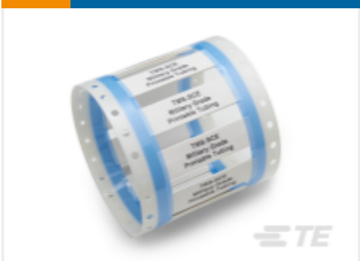
TE 产品编号344283-000 TMS-SCE 军规级套管
