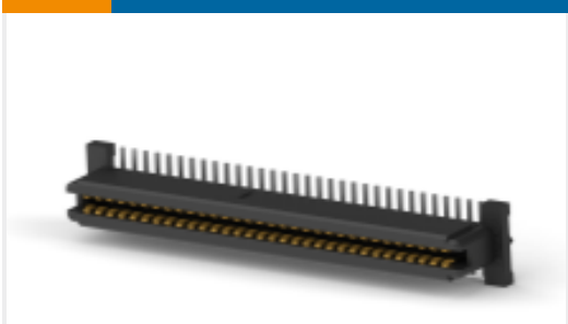
TE 产品编号5146893-2 自由高度插座连接器：板对板，垂直，84，1mm
