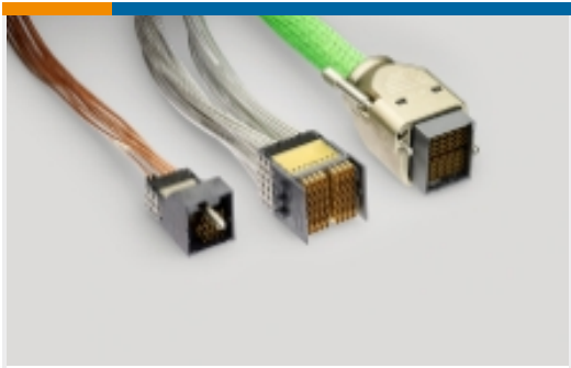
高速背板光缆组件(16)
