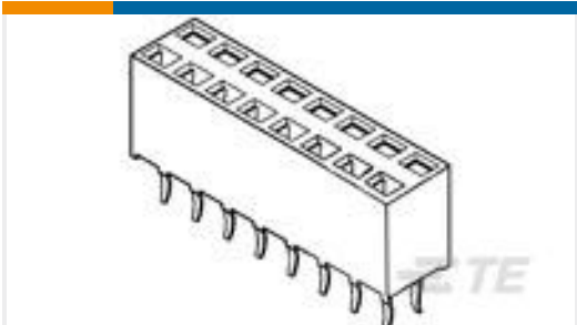
TE 产品编号215307-2 2X2P HV100 REC CON. TE, 7.0MM
