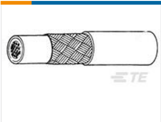
TE 产品编号3310063004 55A1111-24-9-9
