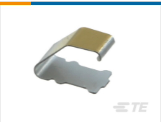
TE 产品编号1734300-1 SHIELD FINGER 3025-Z1-T
