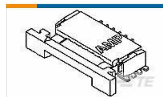
TE 产品编号1-84952-7 1MM FPC HORZ.BTTM CONT.ASS.17P
