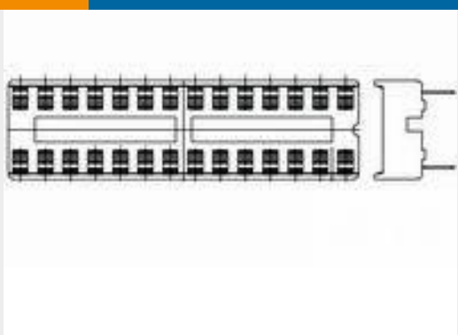
TE 产品编号1-2199298-8 24P,DIP SKT,300 CL,LDR,PB FREE
