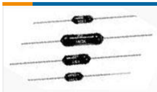
TE 产品编号1-1879663-3 H8 143R 0.1% 15PPM
