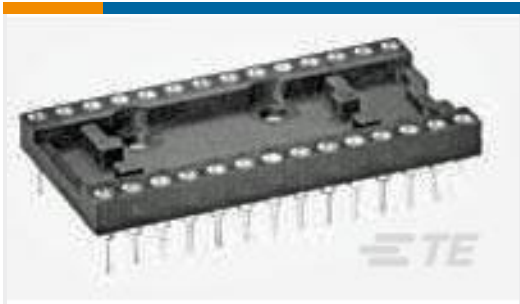
TE 产品编号1571551-4 516-AG12D-ES-LF=500 DIP,SN/SN
