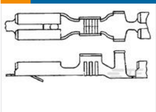
TE 产品编号170042-2 FF 110 REC 20-16AWG TPBR
