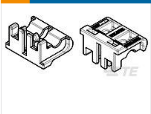
TE 产品编号1939393-1 0.64/2.3mm SEALED CLIP
