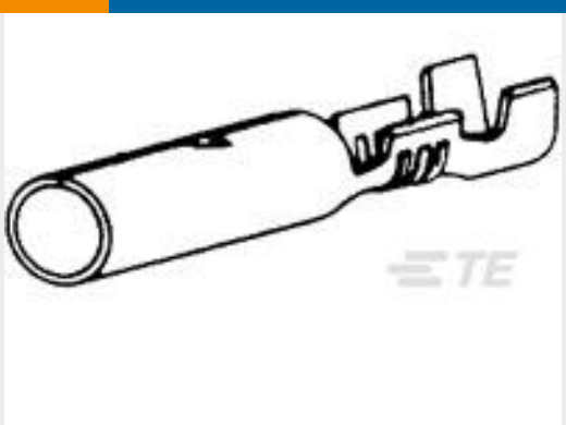
TE 产品编号42531-3 180 SHPL REC 20-16 016PHBZ
