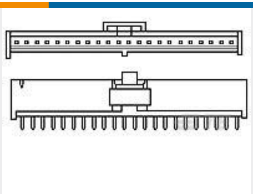
TE 产品编号3-1888291-3 FPH-2021G=FLXPAC HDR P 20 ST L
