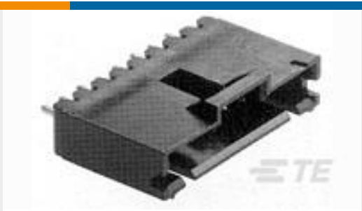
TE 产品编号 5-104362-1 02 MTE HDR SRST LATCH W/HLDWN
