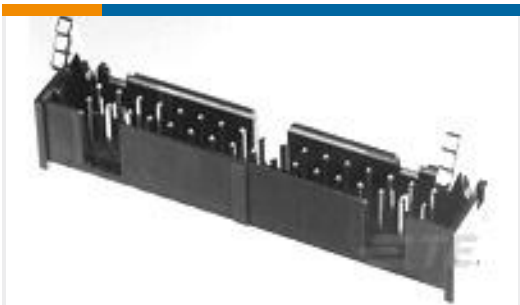
TE 产品编号1-1761606-0 IDC LOW PRO HDR 30P VERT LG LA
