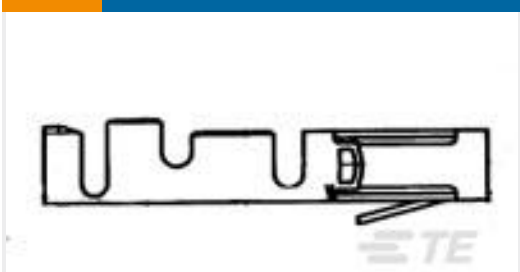
TE 产品编号181270-2 MOD II CONTACT L.P.
