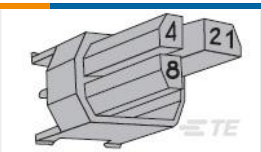
TE 产品编号102154-4 020 UNIV HDR SP 4S 30DP STD
