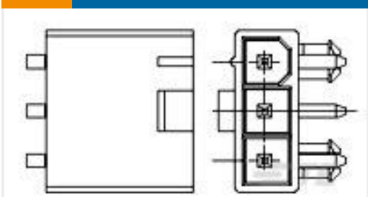
TE 产品编号2029150-5 5P R/A HDR VAL-U-LOK V2 W/P
