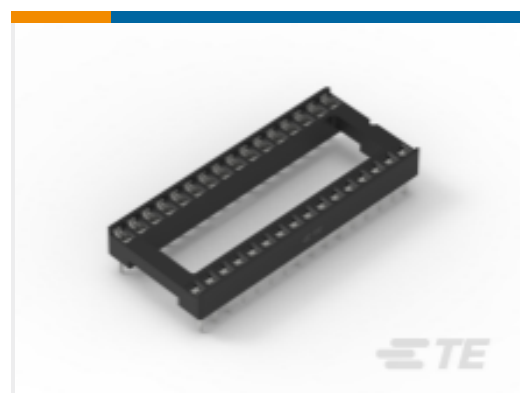
TE 产品编号 1-2199300-2 32P,DIP SKT,600 CL,OTC,PB FREE
