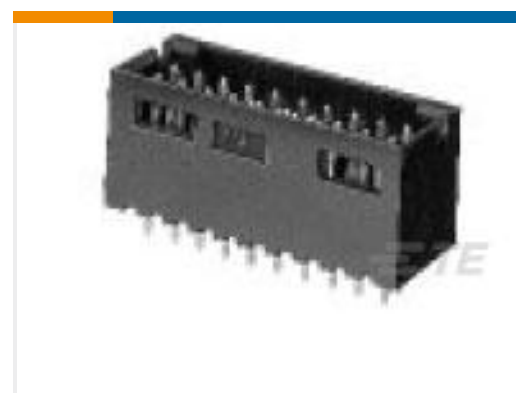
TE 产品编号 102618-6 16 MODII HDR DRST SHRD .100CL
