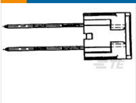
TE 产品编号917894-1 2.5 S.D.L STD V 2P HDR ON/TAPE
