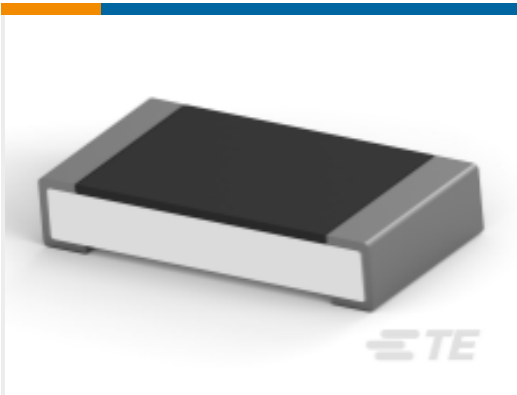
TE 产品编号4-2176392-5 RQ 1206 383K 0.1% 10PPM 5K RL
