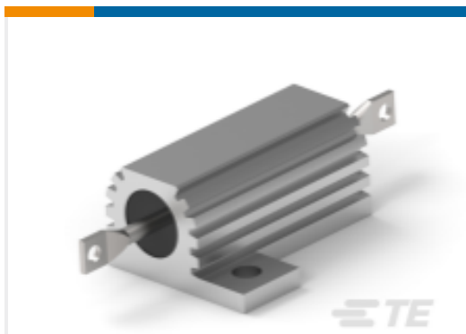
TE 产品编号1-1879073-0 功率电阻器：铝壳体，75 瓦特
