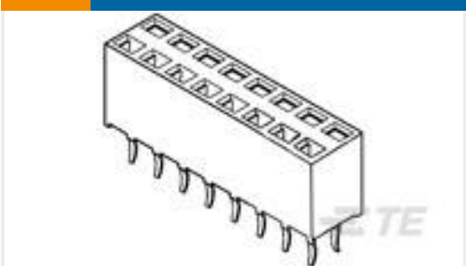
TE 产品编号1-215307-4 2X14P HV100 REC CON. TE, 7.0MM
