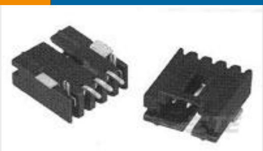
TE 产品编号 5-147278-8 09 MTE HDR SRRA SFMNT .100CL
