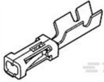
TE 产品编号 87666-2 MOD IV RECP PLTD 30 SEL
