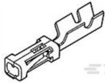
TE 产品编号 2-87523-3 MOD IV RECP PLTD 15 DPLX
