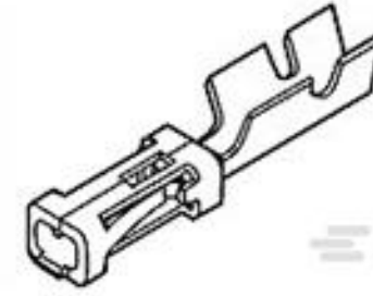
TE 产品编号 6-87756-2 MOD IV RECP PLTD 15 DPLX LF
