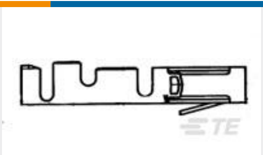
TE 产品编号141098-6 MOD-4 REC.CONTACT
