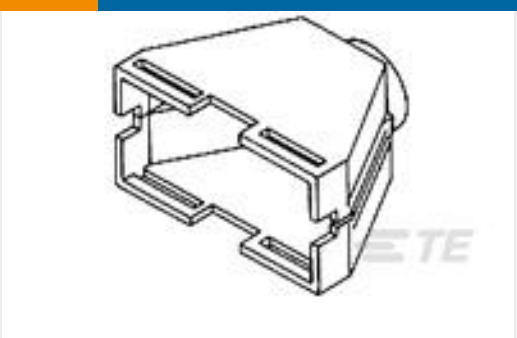
TE 产品编号1-480594-9 36P STR/REL HNGD BLK
