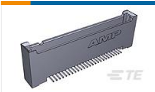
TE 产品编号146839-1 50 MC HDR VERT SMTW/BRD LOC
