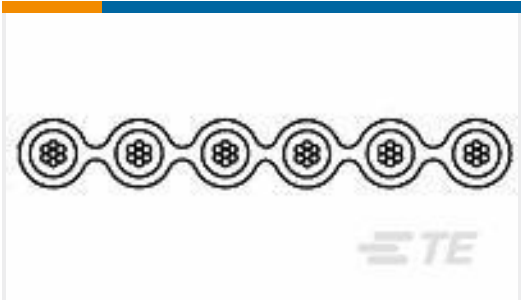
TE 产品编号1-167019-0 10P. RIBBCBL 28AWG P1.27
