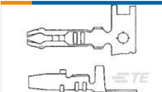
TE 产品编号170338-1 AMP-IN 22-18 AWG
