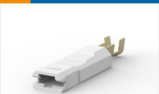
TE 产品编号5-520963-1 ULTRA POD：直形，母端组件，无镀 层，0.250 英寸
