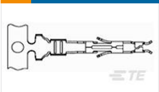
TE 产品编号 1934182-1 UPC Receptacle Contact
