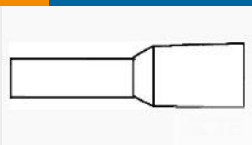
TE 产品编号2-966067-4 ADERENDHUELSE N RT
