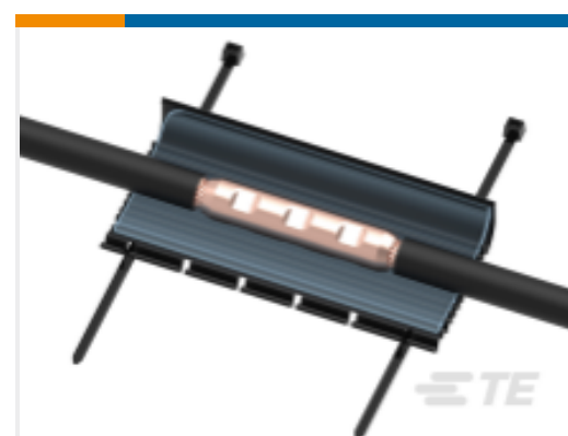
TE 产品编号 E86269-000 GELWRAP-33/10-200(B6)
