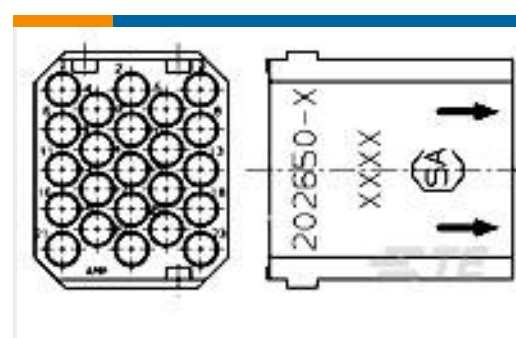
TE 产品编号202650-2 PIN MODULE, 23 POSN, G-SERIES
