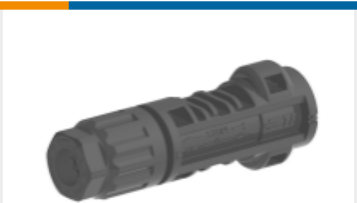
TE 产品编号2-2270024-1 SOLARLOK PV4-S 直流压接连接器
